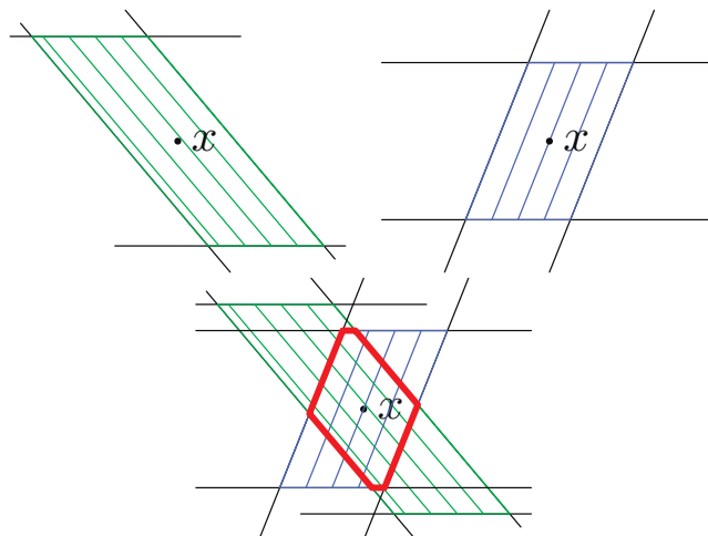
Рис. 12. Пересечение окрестностей
