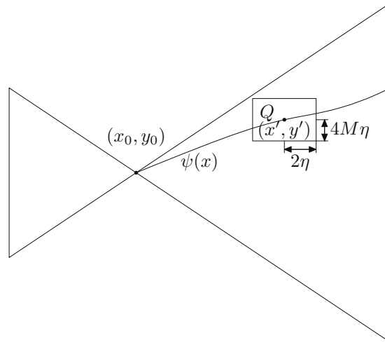
Рис. 16. Прямоугольник Q
